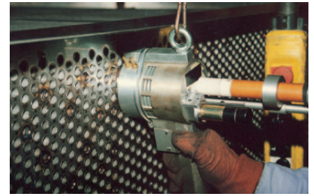
Orbitalschweißungen für komplette Gasdichtheit
